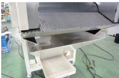
■テール部仕様 (逆回転して研磨剤を回収します)
