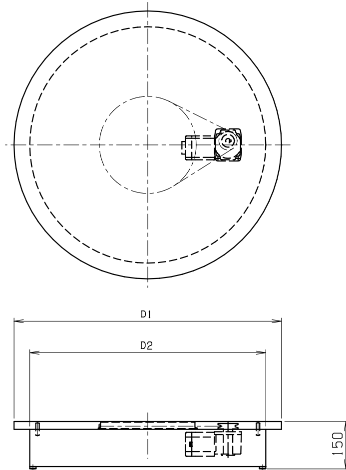
フラットタイプ RT-VB-F型
